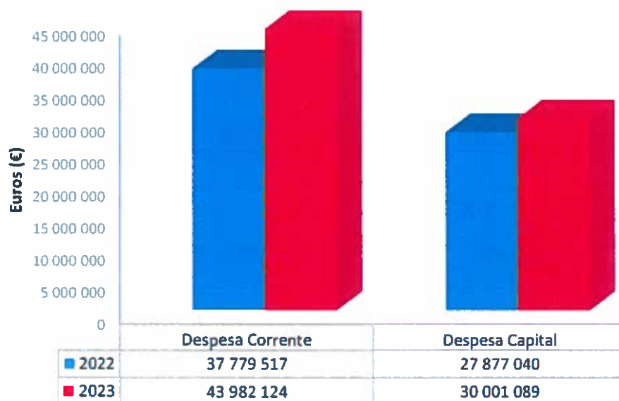
Gráfico 4 - Despesa 2022 vs 2023
